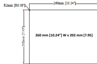
Cutout Dimensions
