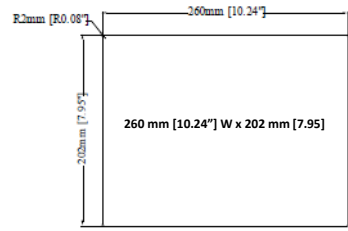
Cutout Dimensions
